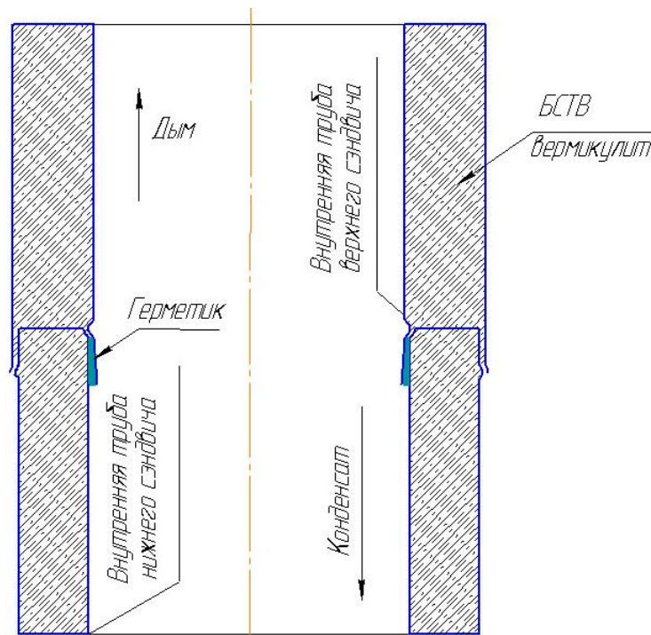
Рис. 3. Схема сборки двухконтурной трубы («сэндвич».) (Разрез по вертикальной оси «сэндвича».)
