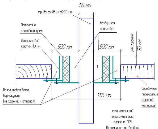
Б). При одноконтурной трубе.
